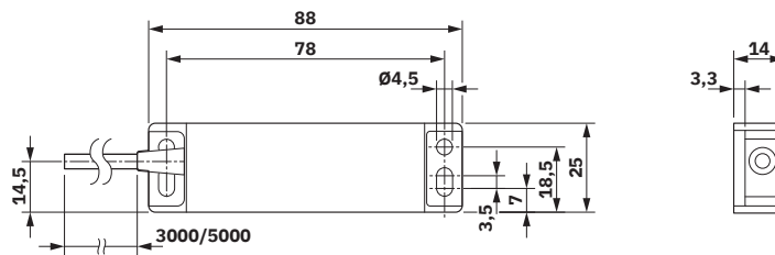
Maßzeichnung
