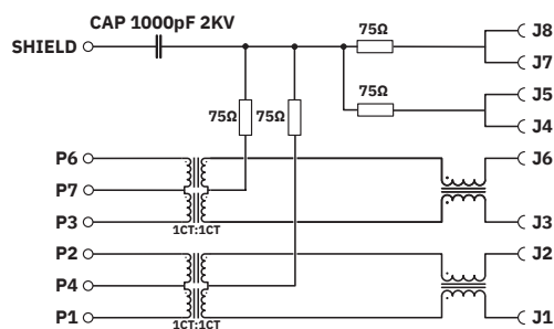
Schaltplan
