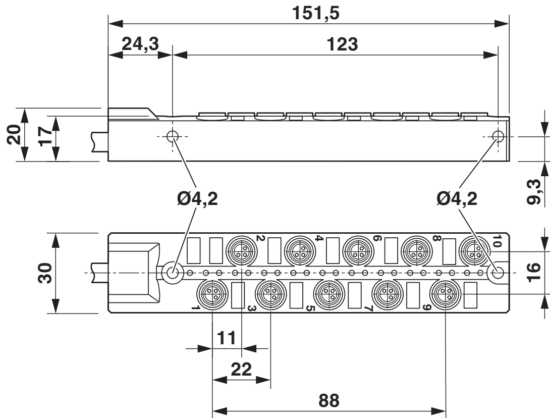
Maßzeichnung
