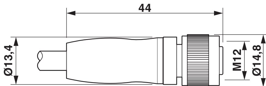
Maßzeichnung
