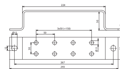
Maßbild ES 2X4 ASB11 STTZN
