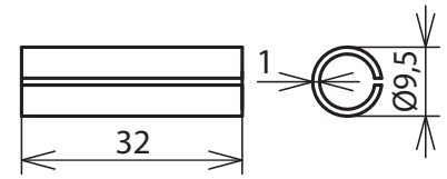
Maßbild CUPAH GL Q35 L32 AL CU
