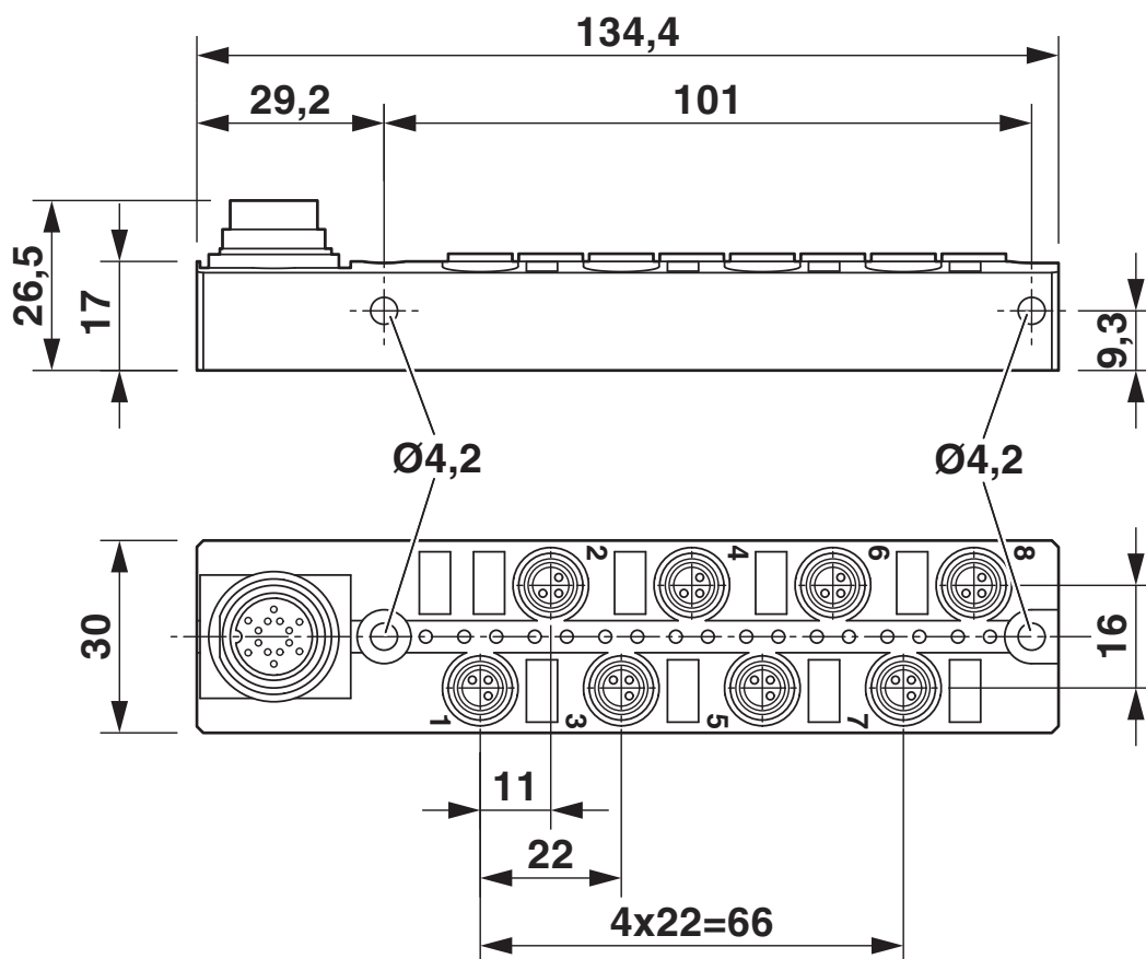
Dessin coté
