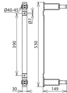
Maßbild HV P ST D40 45
