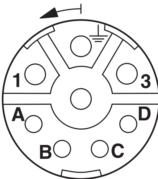
Dessin schématique
