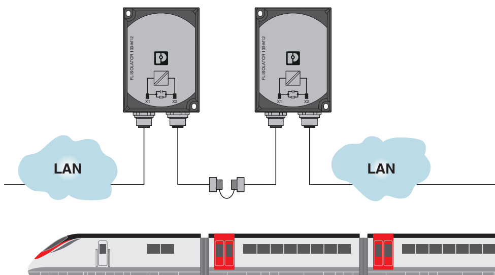
Dessin schématique
