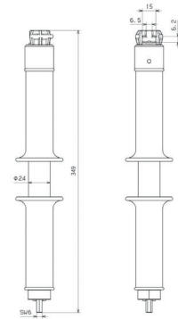
Maßbild EG 00 4A VI
