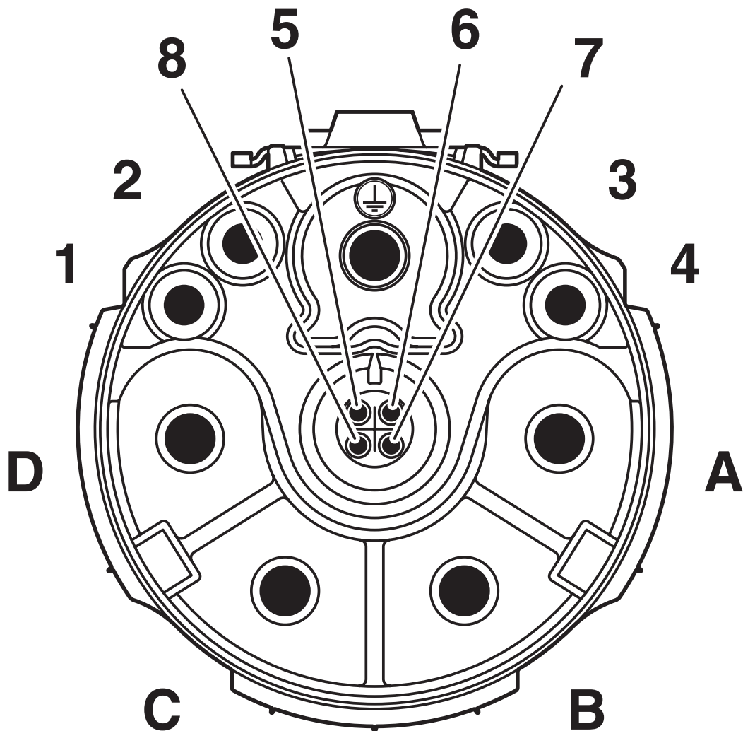
Schemazeichnung
