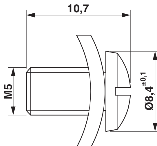
Dessin coté
