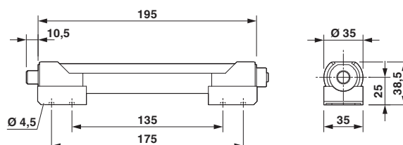
Dessin coté
