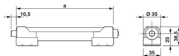
Dessin coté
