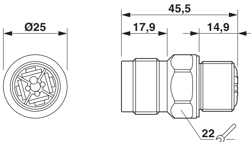
Maßzeichnung
