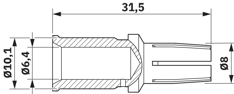
Maßzeichnung
