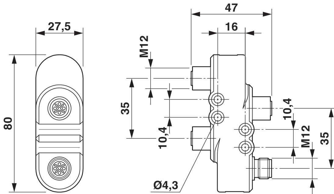
Répartiteur en H M12
