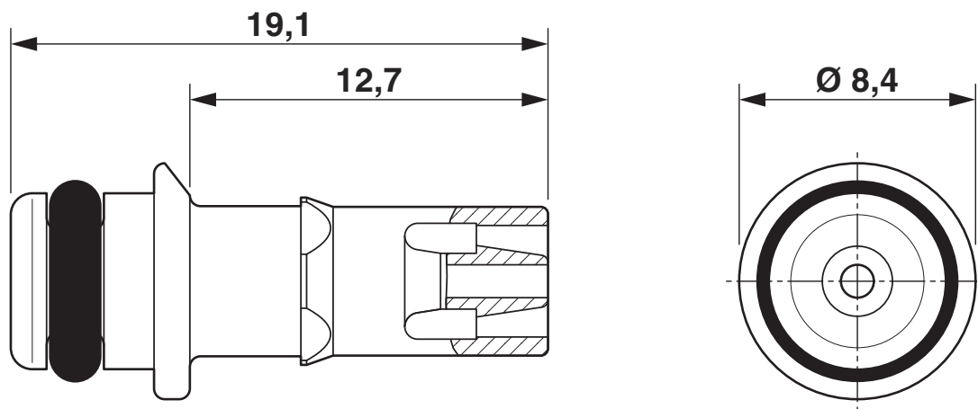
Maßzeichnung
