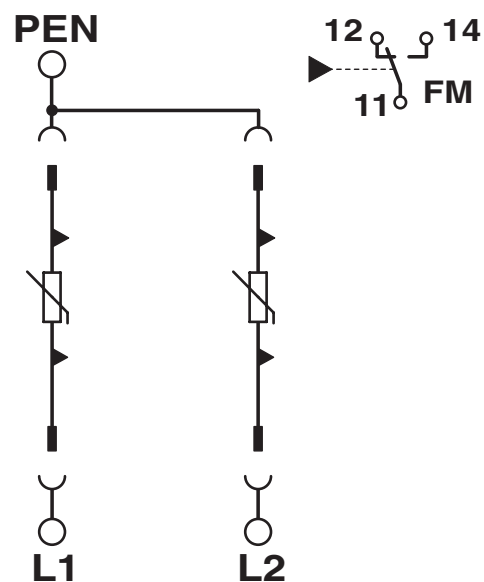
Schaltplan
