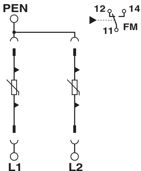
Diagrama eléctrico
