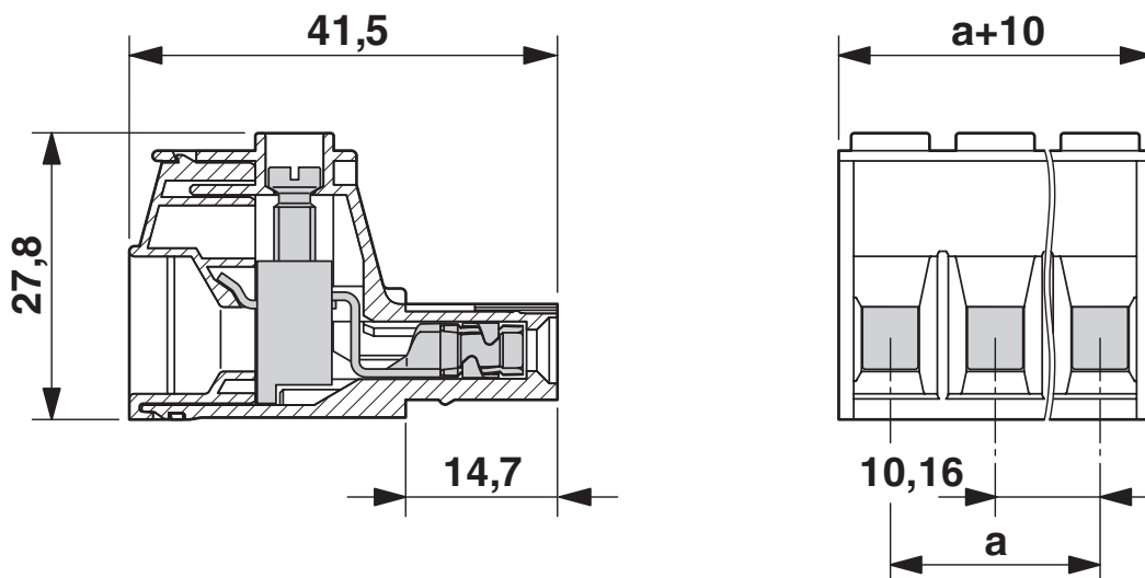
Dessin coté
