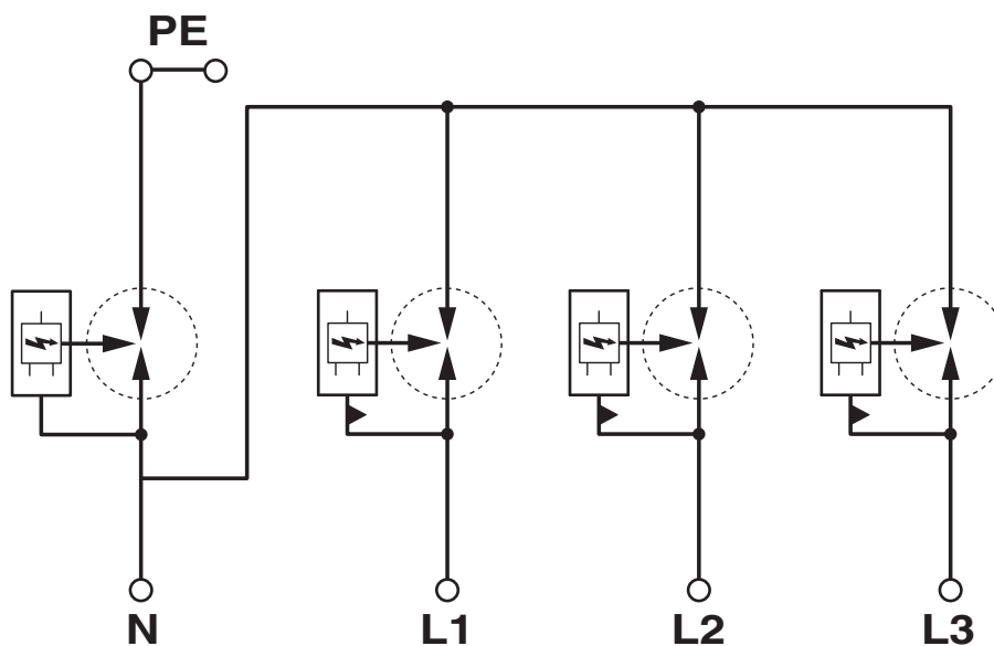
Diagrama eléctrico
