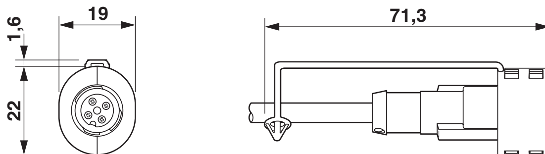
Connecteur femelle montée avec EXCLIP
