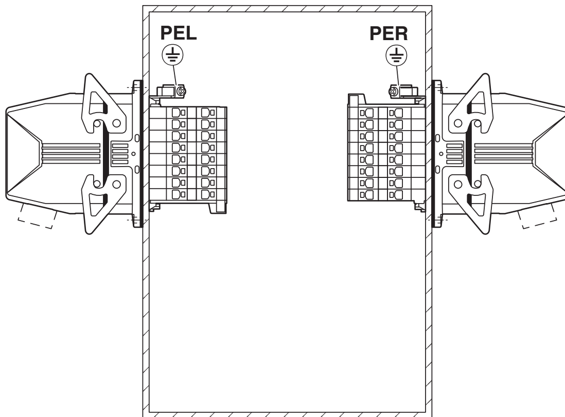
Applikationszeichnung
