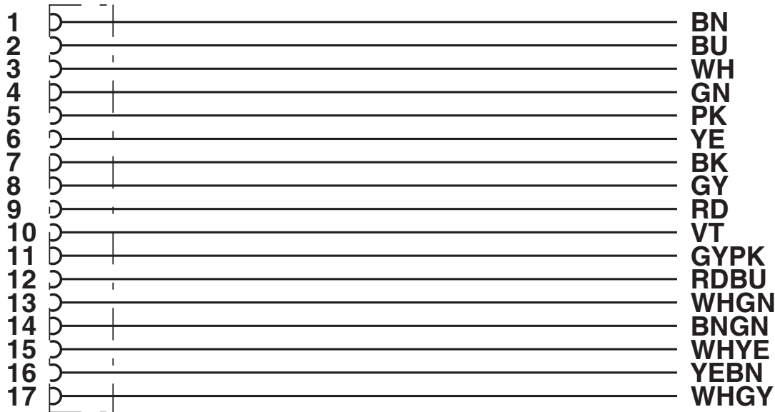
Diagrama eléctrico
