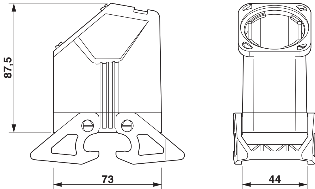
Maßzeichnung
