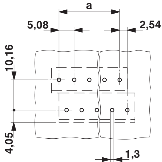
Bohrplan/Lötpadgeometrie
