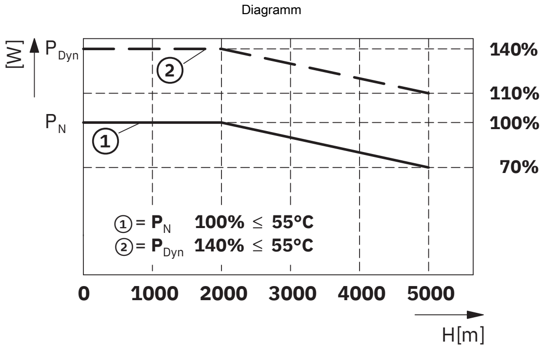
Höhenabhängiges Derating
