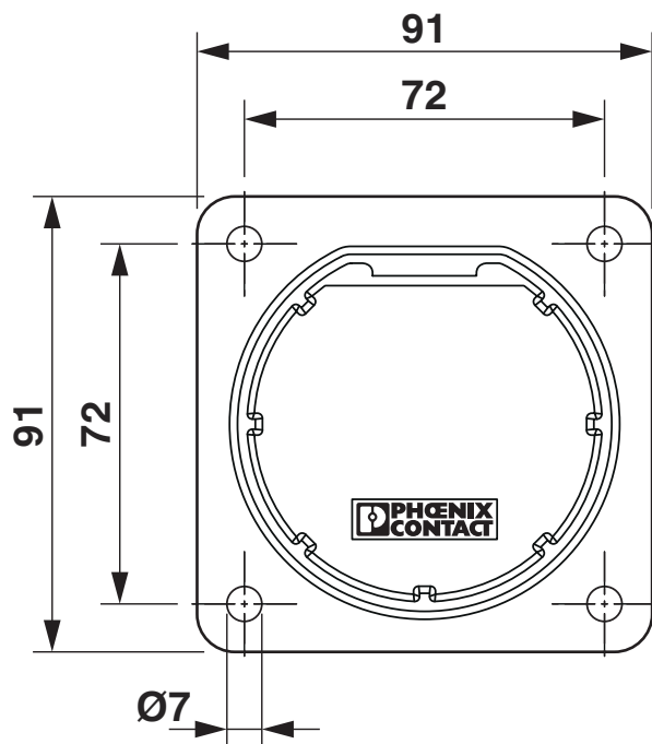
Maßzeichnung
