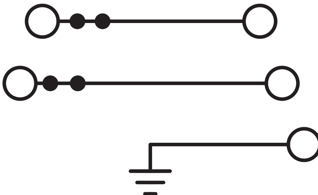
Diagrama eléctrico
