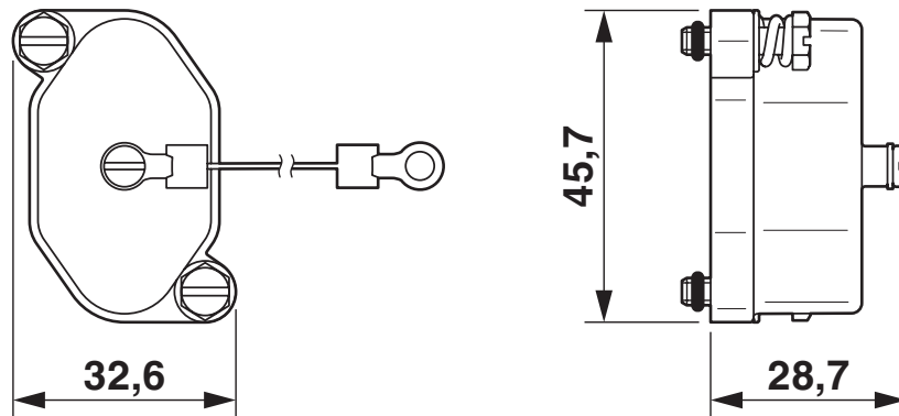
Maßzeichnung
