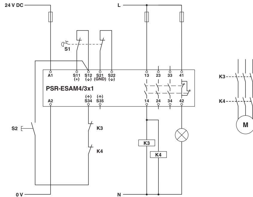
Diagrama eléctrico
