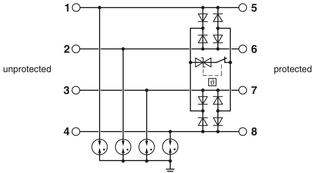
Diagrama eléctrico
