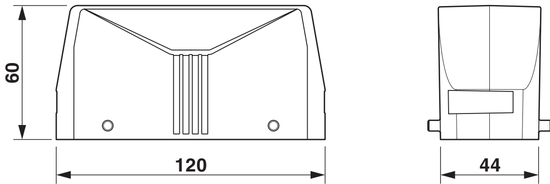
Maßzeichnung
