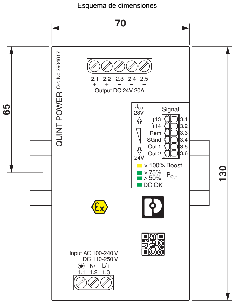
Dimensiones del dispositivo (medidas en mm)
