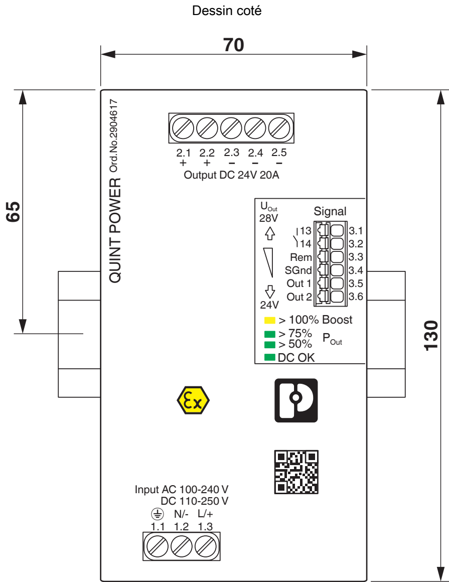
Encombrement de l'appareil (cotes en mm)
