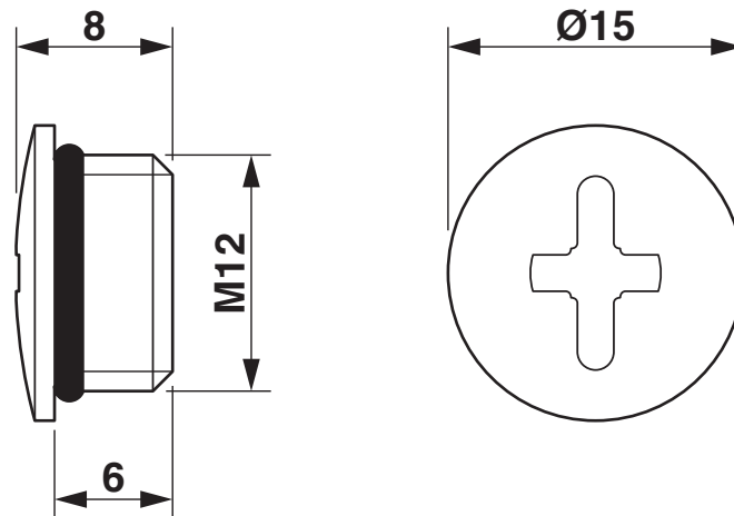
Maßzeichnung
