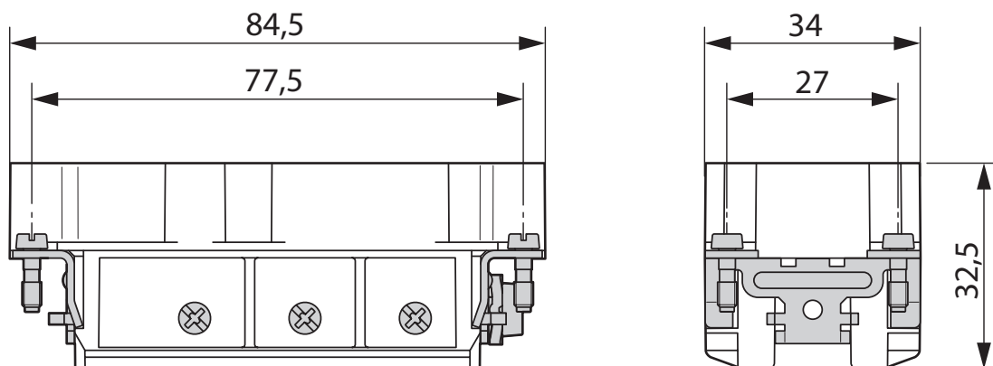
Dessin coté
