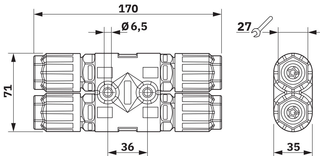
Dessin coté
