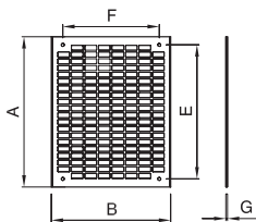
piastre forate in acciaio
