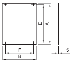
piastre in materiale isolante
