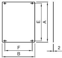
piastre in acciaio
