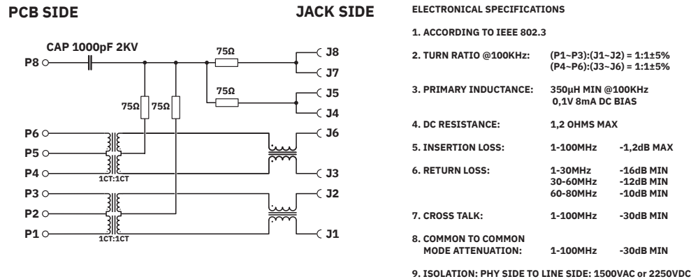
Diagrama eléctrico
