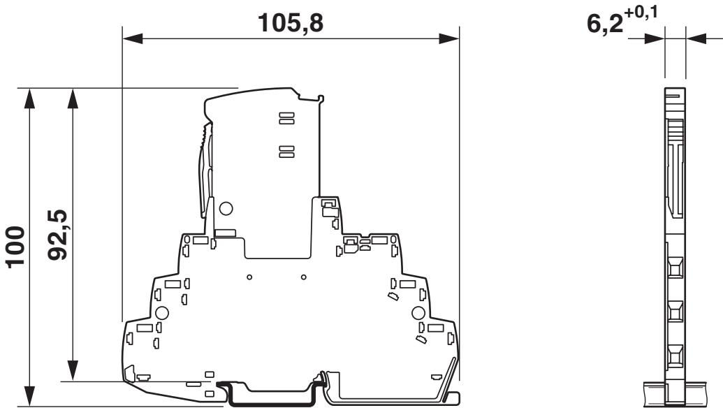
Plano esquemático
