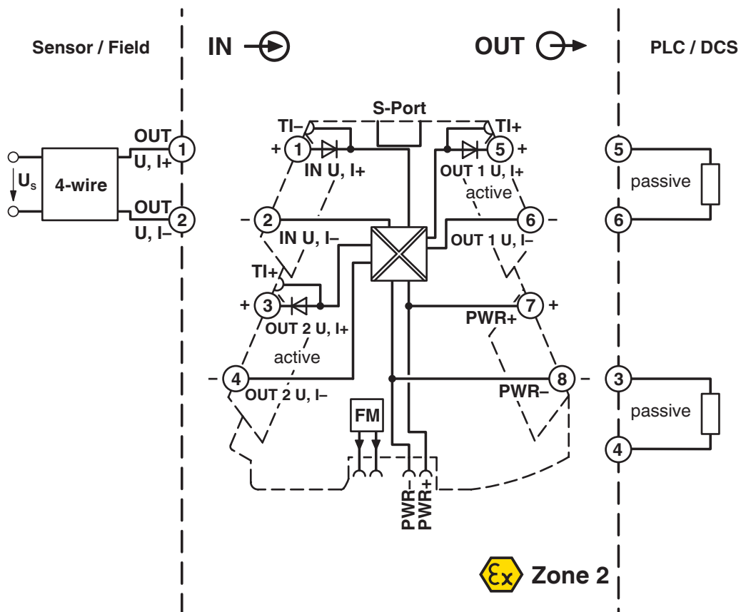
Schéma fonctionnel
