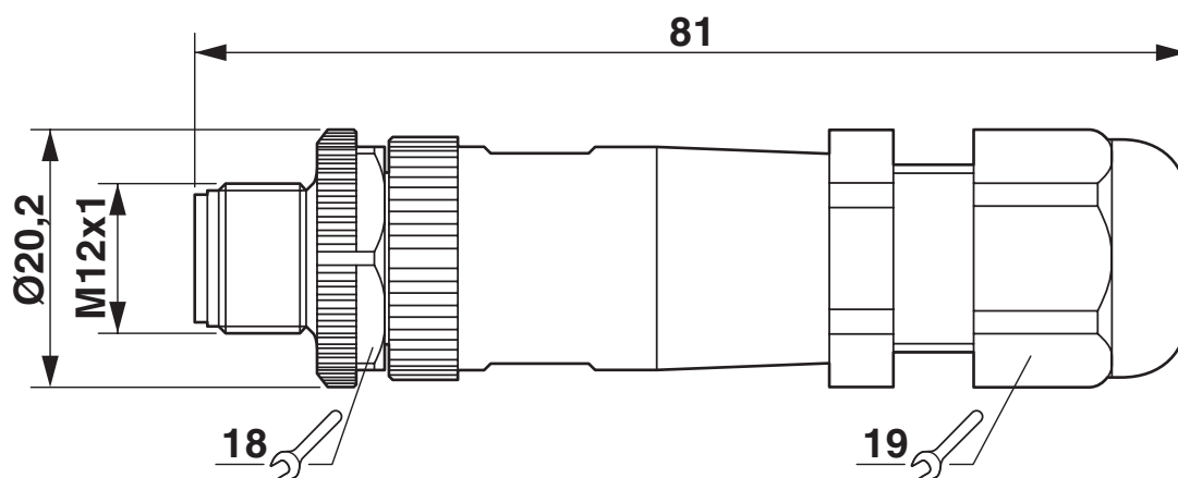
Maßzeichnung
