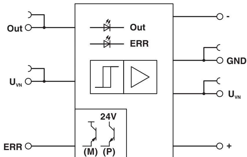
Diagrama eléctrico
