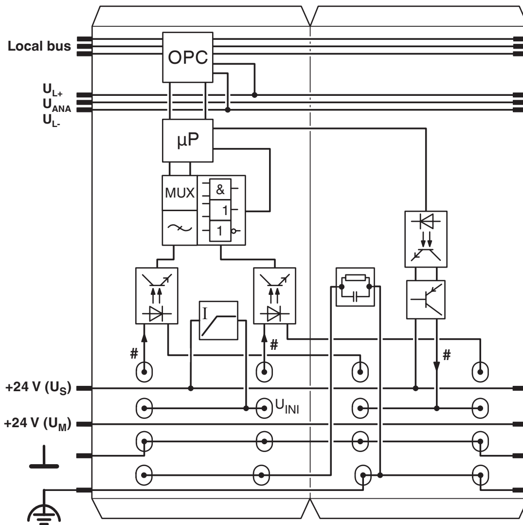
Schéma fonctionnel
