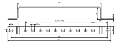
Maßbild ES 10AP 11X11 V2A
