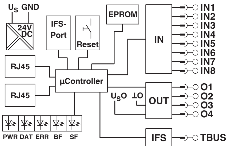
Blockschaltbild
