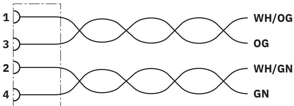
Ocupación de contactos del conector hembra M12
