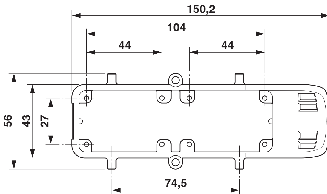
Esquema dimensiones vista desde arriba
